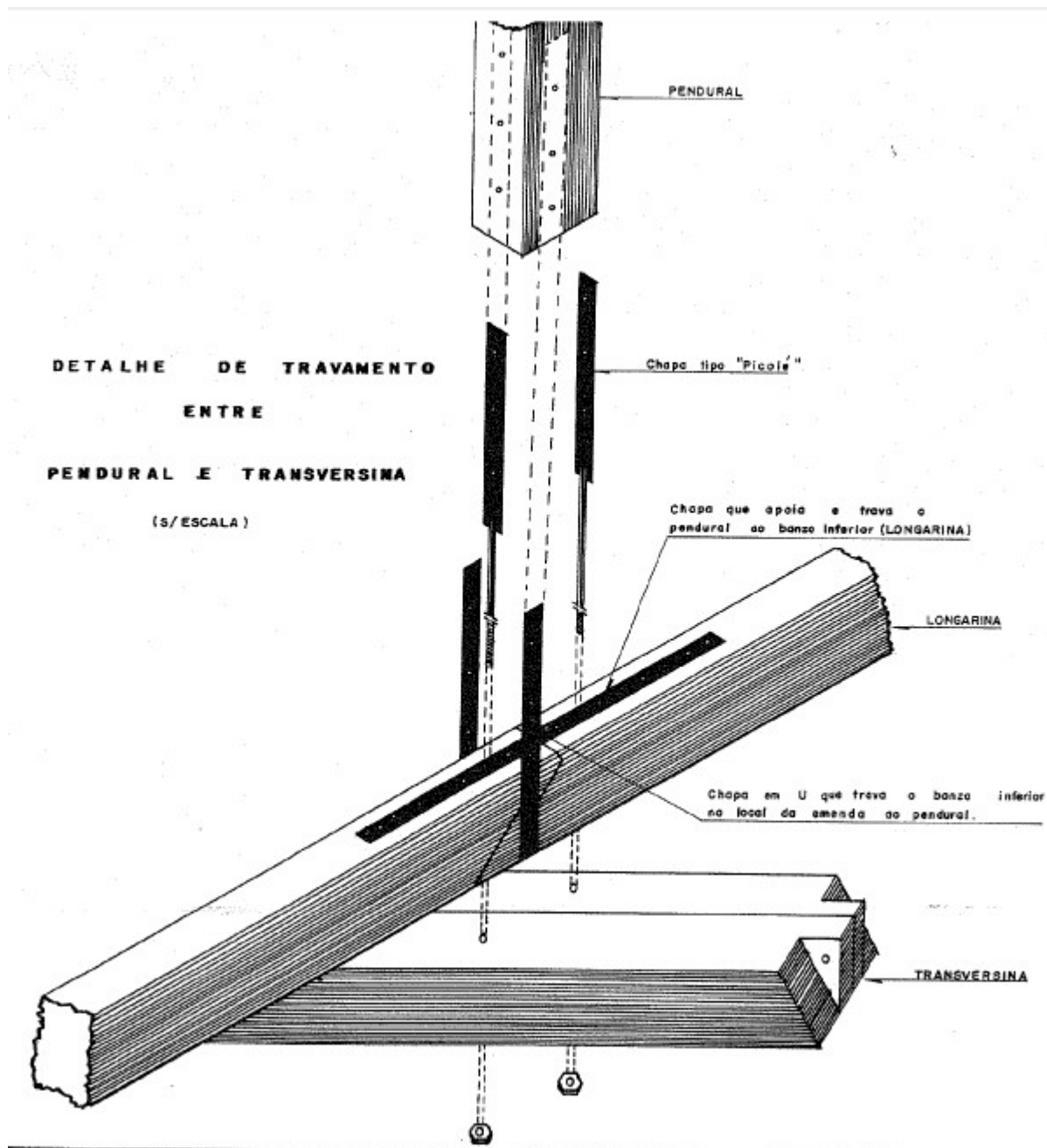
Figura 09: Detalhe de travamento entre pendural e transversina
