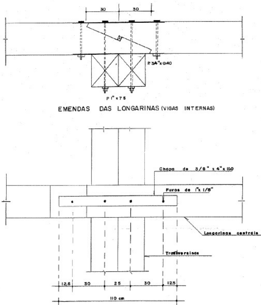
Figura 03: Emenda de vigas
